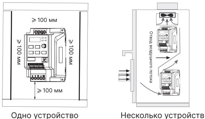
Рисунок 3-1. Схема установки преобразователей частоты
