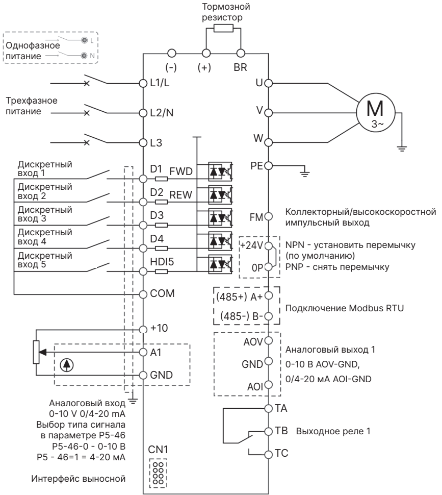
Рисунок 3-3. Схема подключения клемм
