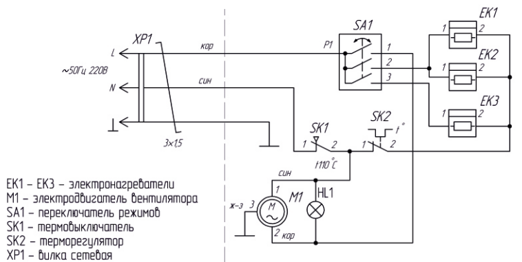
Схема коммутации переключателя SA1
