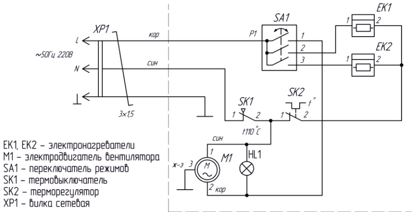
Схема коммутации переключателя SA1
