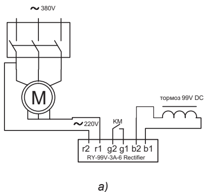
Схема 10. При соединении обмоток в коробке выводов по схеме "звезда", а) - с одним тормозом, б) - с двумя тормозами
