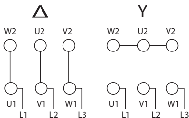
Рисунок А.1.2 - Схема подключения двигателя с соединением фаз обмотки «Δ/Y» (шесть выводных концов)
