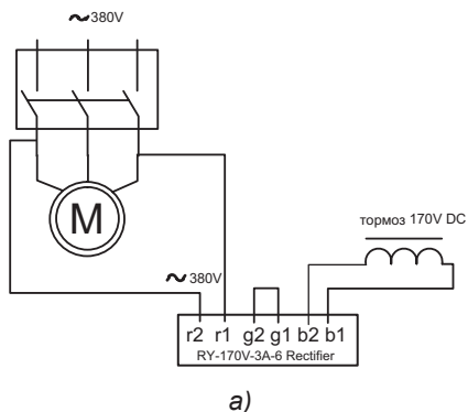
Схема 9. а) - с одним тормозом, б) - с двумя тормозами
