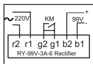
Схема 9. а) - с одним тормозом, б) - с двумя тормозами
