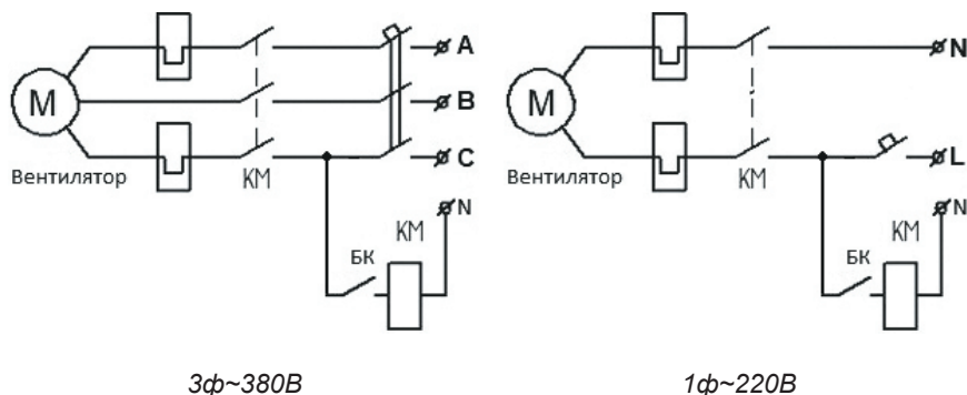
Схемы подключения вентилятора:
