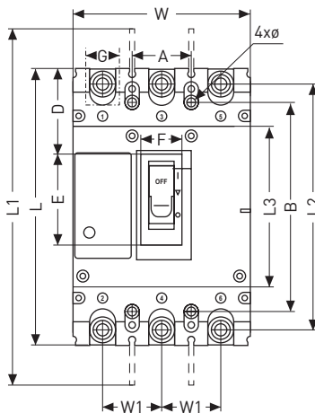
3-х полюсной
