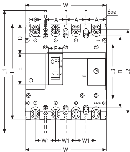
4-х полюсной
