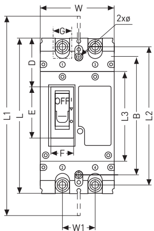
2-х полюсной
