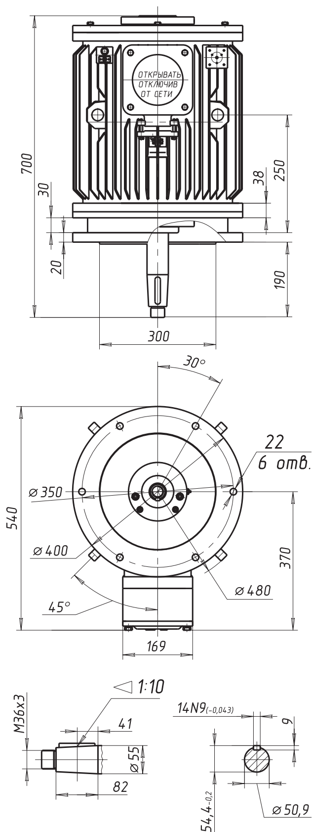
Рисунок 5. ВАСОУ-6,5-12 (Монтажное исполнение IM 3013) Масса - 185 кг
