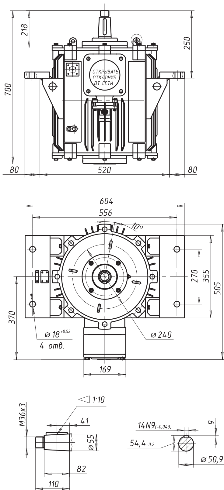
Рисунок 6. ВАСОУ-6,5-12 (Монтажное исполнение IM 9633) Масса - 185 кг
