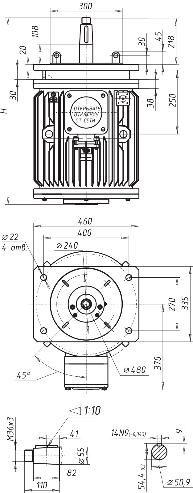
Рисунок 11. ВАСОУ-9 (-13, -15, -18,5) -12 (Монтажное исполнение IM 3033) (с квадратным фланцем)
