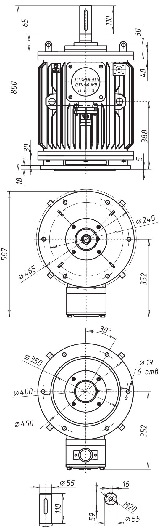
Рисунок 16. ВАСОУ-18,5-12 (Монтажное исполнение IM 3031) Масса - 400 кг
