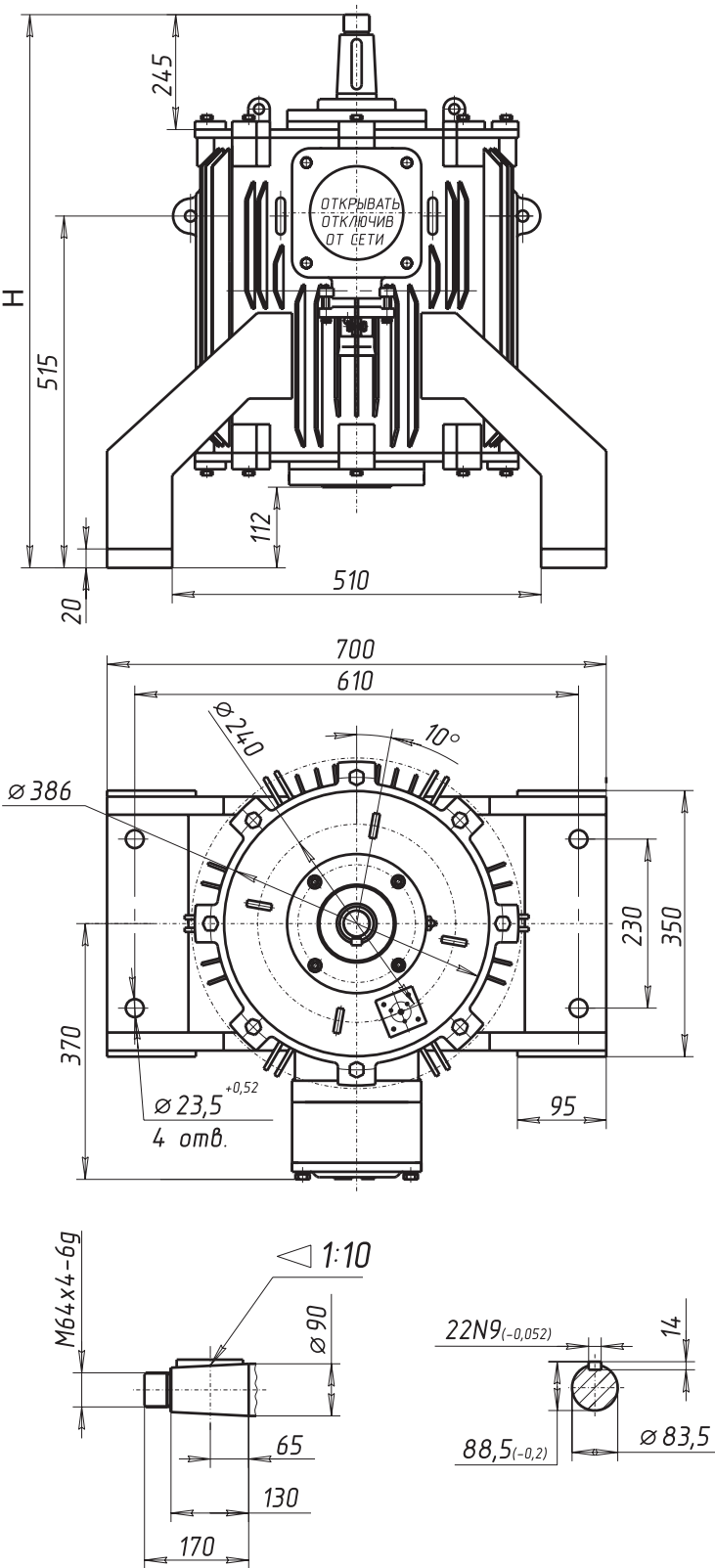
Рисунок 15. ВАСОУ-9 (-13, -15) -12 (Монтажное исполнение IM 9633) (сварные лапы)
