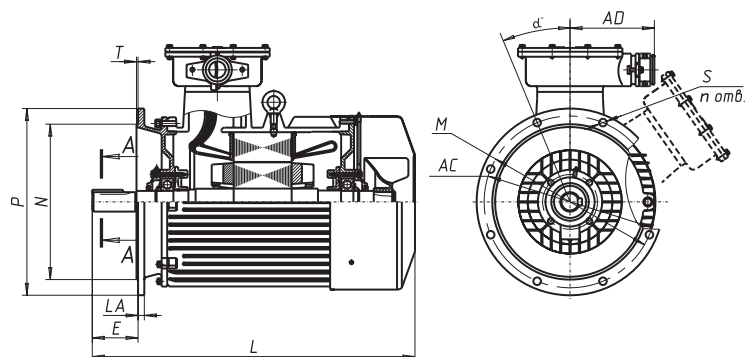
A-A исполнение 1
