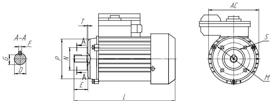
Исполнение IM 3681/B14
