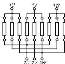
Схема обмотки
